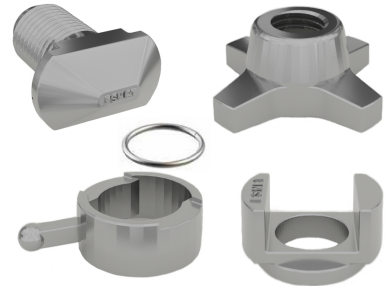
Containerschloss inneres Set 52 mm
