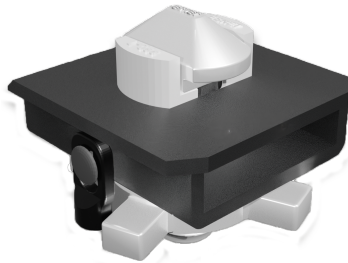
Containerschloss Nschmaler Typ 52mm
